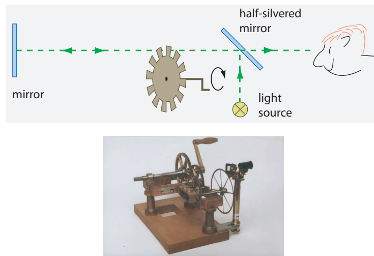
FIGURE 134 Fizeau's set-up to measure the speed of light (© AG Didaktik und Geschichte der Physik, Universität Oldenburg)
