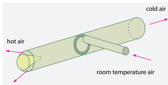
FIGURE 123 The Wirbelrohr or Ranque–Hilsch vortex tube
